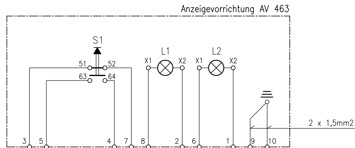
Elektrisches Schema für Bremsanzeige AV 463:
